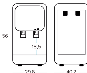
DIMENSIONES (cm)
