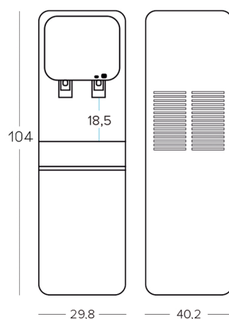
DIMENSIONES (cm)
